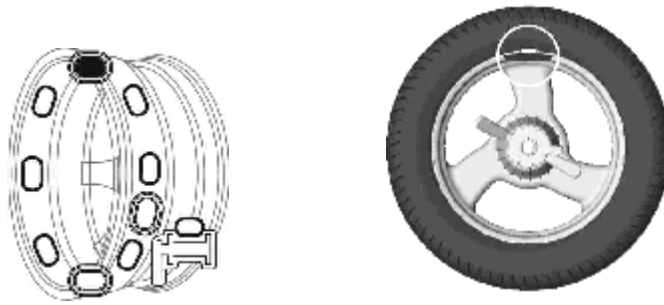
Рисунок 6.3 – Груз установлен в положение «12 часов»
