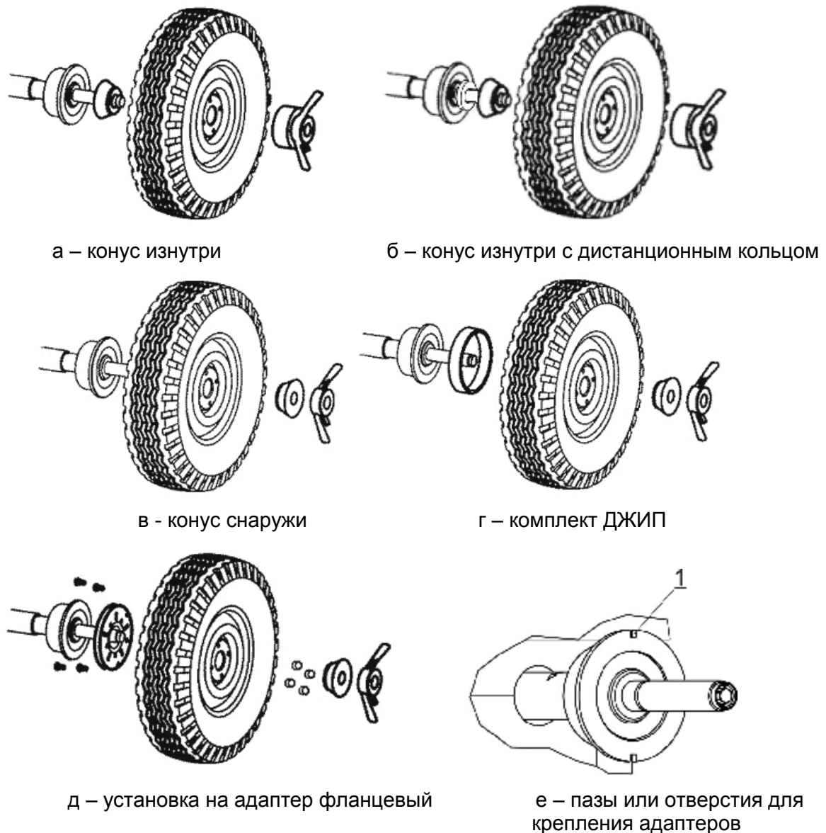
Рисунок 5.1 – Установка колеса
